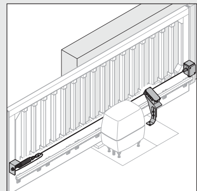
SKS-Schiebetor
